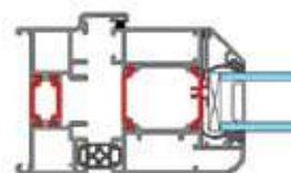
Jamb Detail
